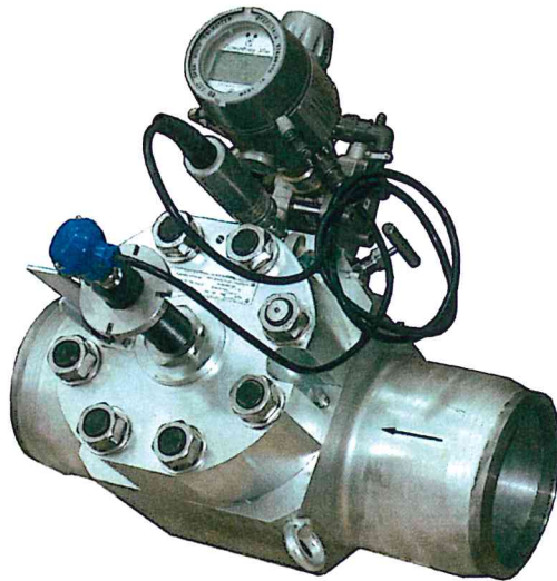
б) Расходомер газа «ГиперФлоу» КРАУ2.833.006-01
